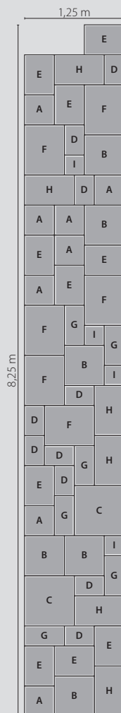
Weg mit einer Breite von 125 cm Verlegung einer Palette mit 58 Stück
