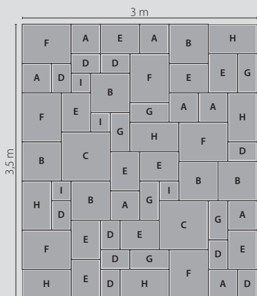
Fläche 3,00 x 3,50 m Verlegung einer Palette mit 58 Stück
