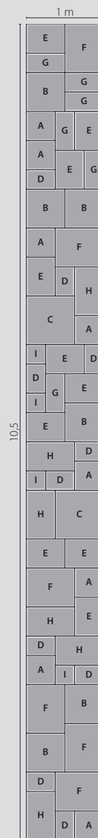
Weg mit einer Breite von 100 cm Verlegung einer Palette mit 58 Stück
