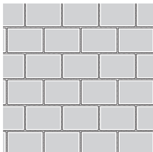
Beispiel 2 (Läuferverband) maschinell verlegbar
